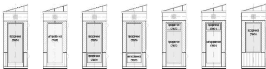
варианты остекления павильонов:
