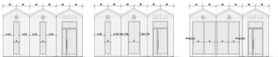
пример павильона с различными вариантами остекления и простенков:
